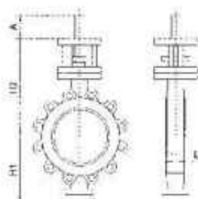
Lug type
