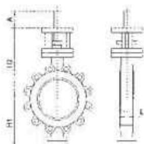
Lug type
